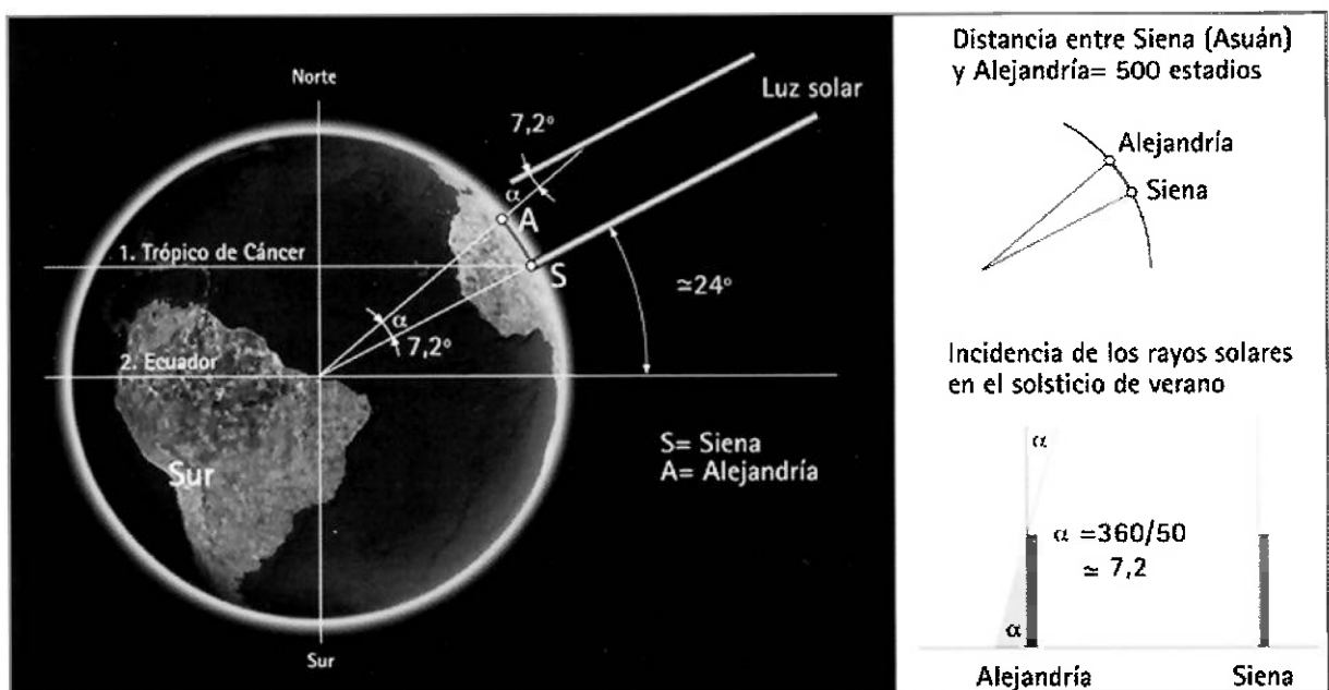
Cálculo de la circunferencia terrestre por Eratóstenes
